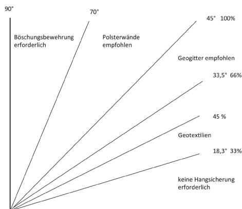
Abb.3.3: Böschungneigung und Verfahren zur Hangsicherung (nach Zimmermann 2009)
