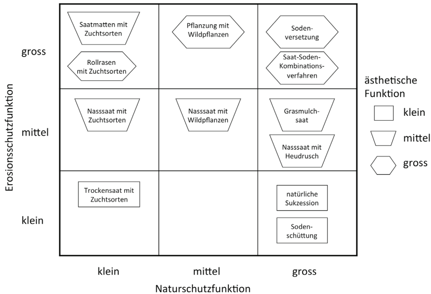
Abb.6.1: Vergleich wichtiger Begrünungsverfahren in Bezug auf Erosionsschutzfunktion, Naturschutzfunktion und ästhetischer Funktion.
