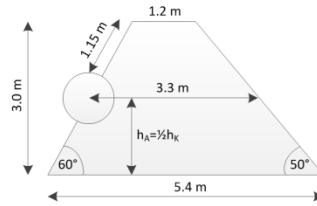
Einschlag auf halber Dammhöhe
