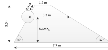
Einschlag mit Freibord halber Blockdurchmesser
