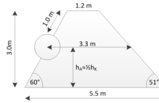
Einschlag mit Freibord Blockdurchmesser
